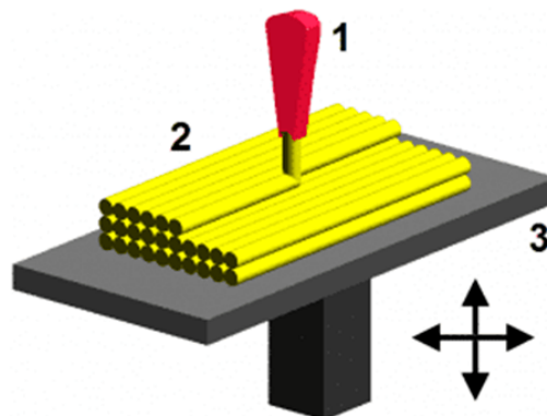
Figura 4: Esquemático processo FDM camada por camada
